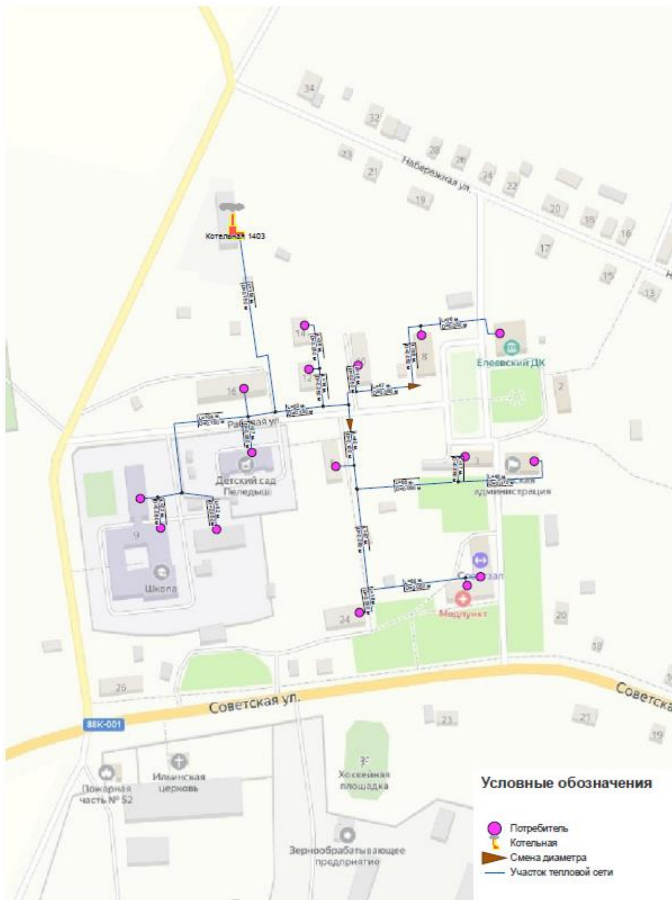
Приложение 1 – Схема тепловой сети с. Елево.
