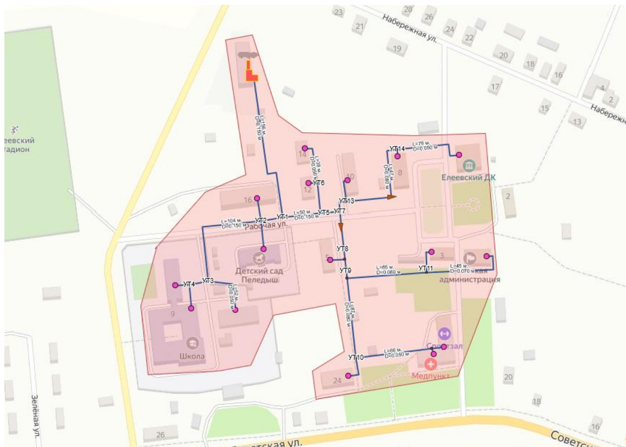
Рисунок 4 – Зоны действия Котельной с. Елеево
