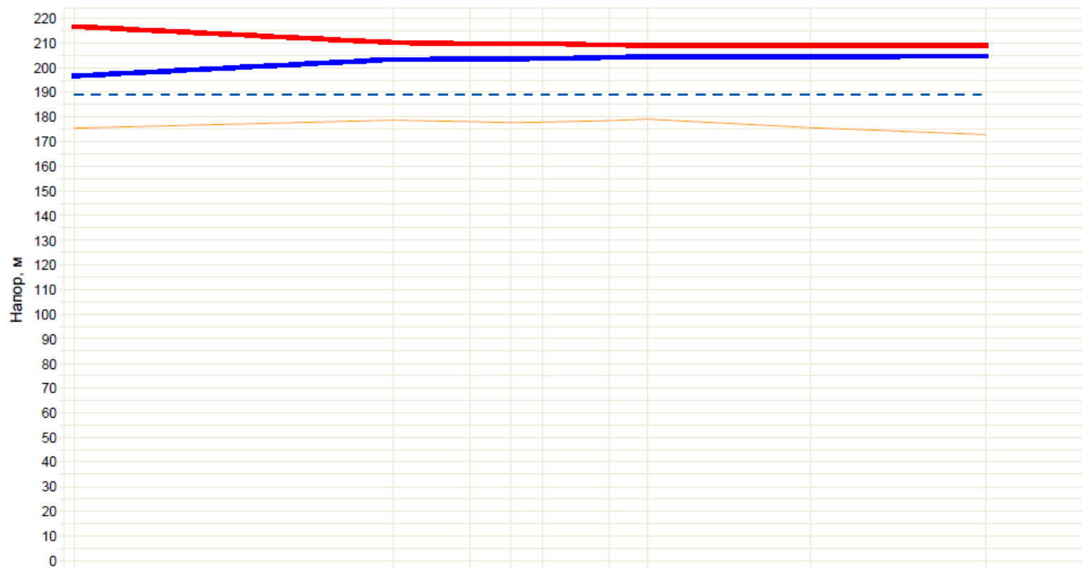
Пьезометрический график от «Котельная 1403» до «Админ. здание»
